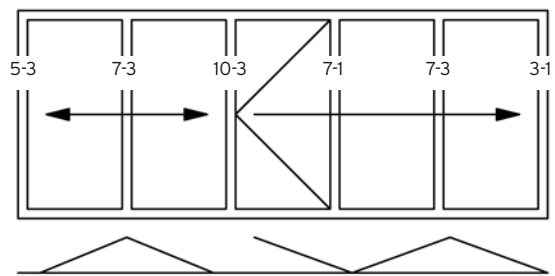
A - 2LR 3R
